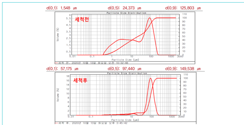
〈그림 3〉 모래 세척 전후 입경분포
