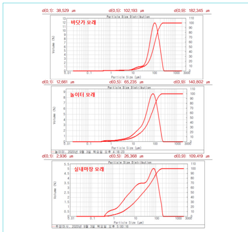
〈그림 2〉 장소별 모래 입경 비교
