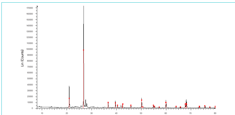
〈표 1〉 벌크(모래)의 결정체 성분 정량분석 결과
